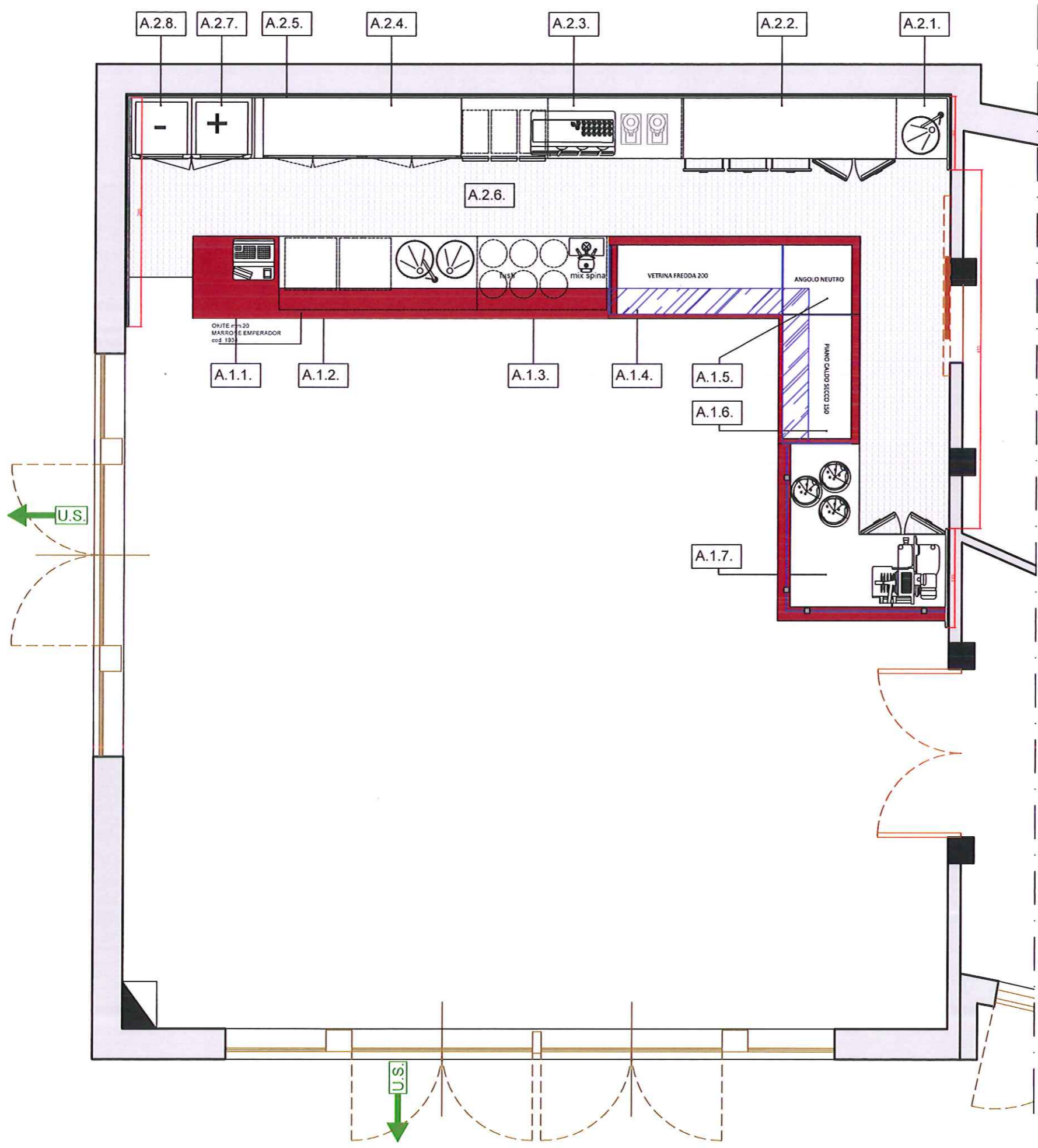
TAV. 02-01 BAR PLANIMETRIA TOTALE
