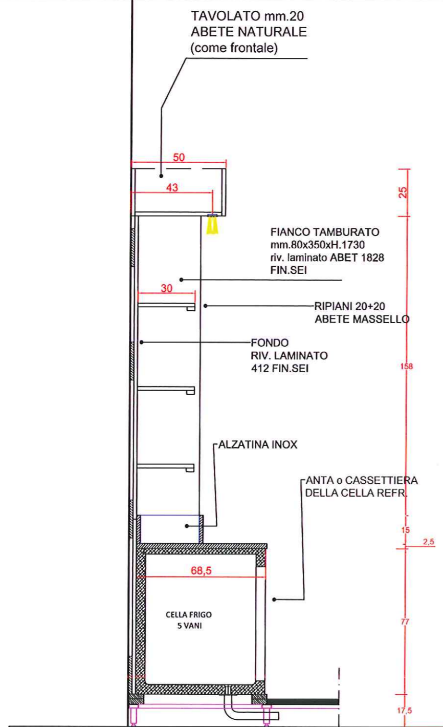
SEZIONE EE': RETRO CELLA REFR.
