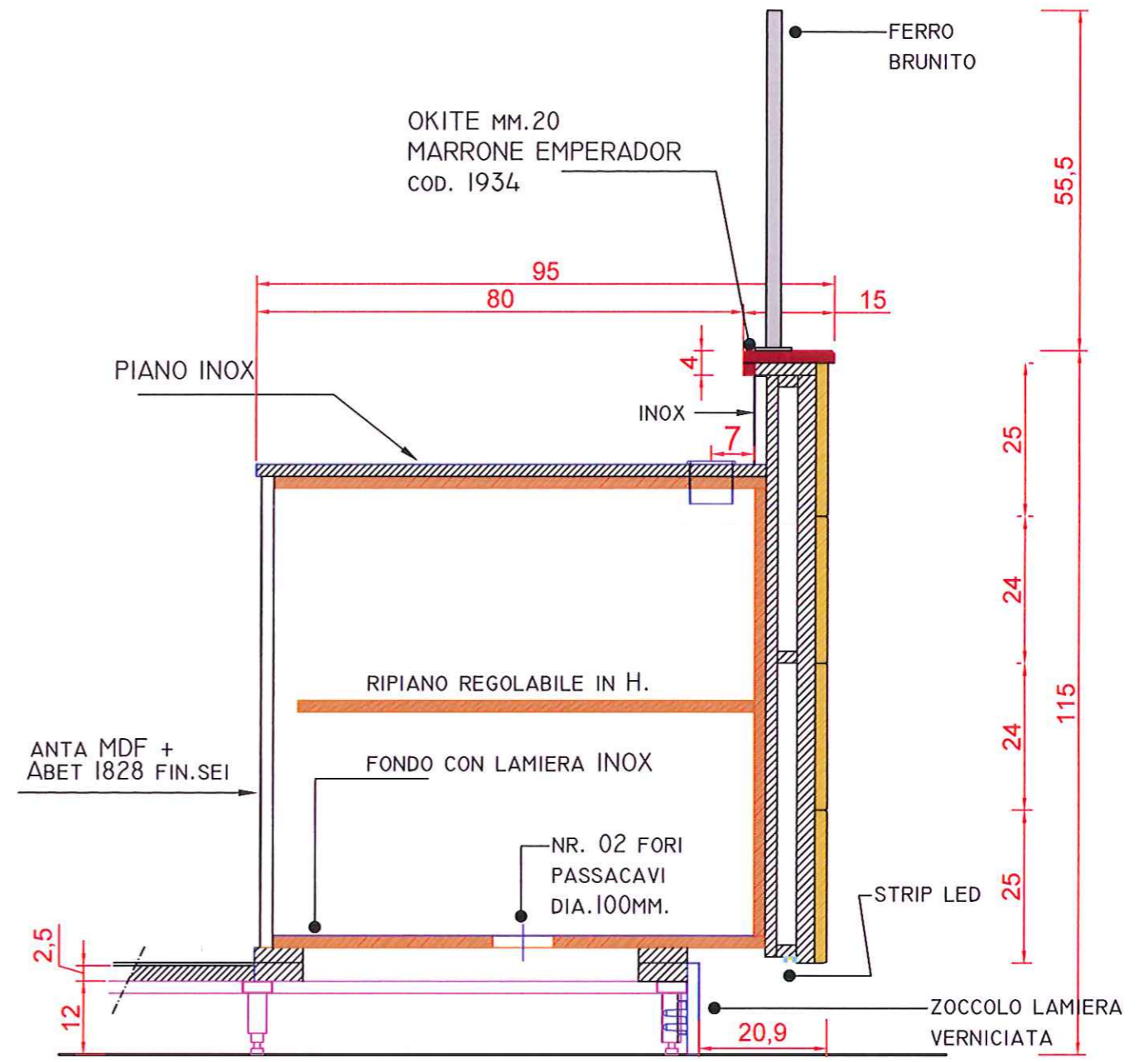
SEZIONE EE': BANCO AFFETTATI
