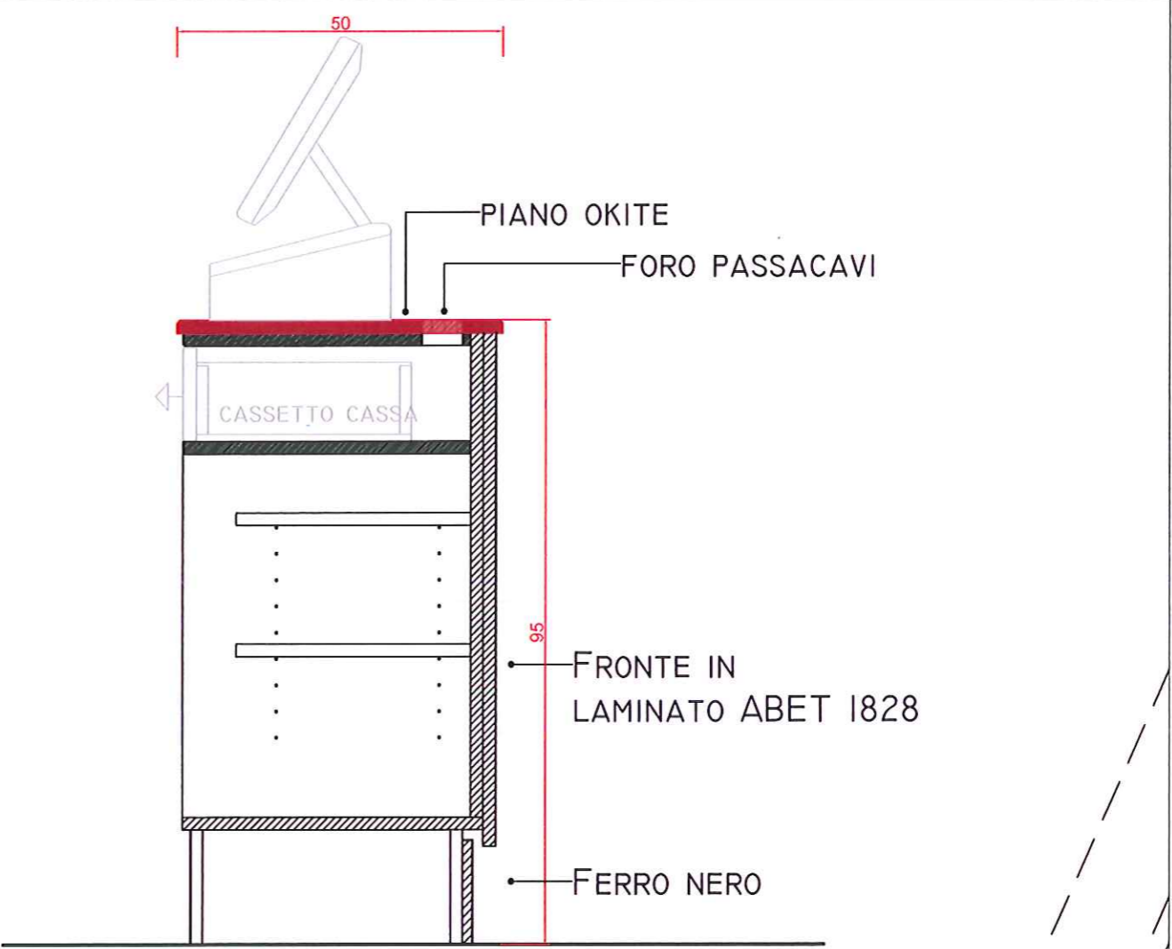
particolare sezione 1:10
