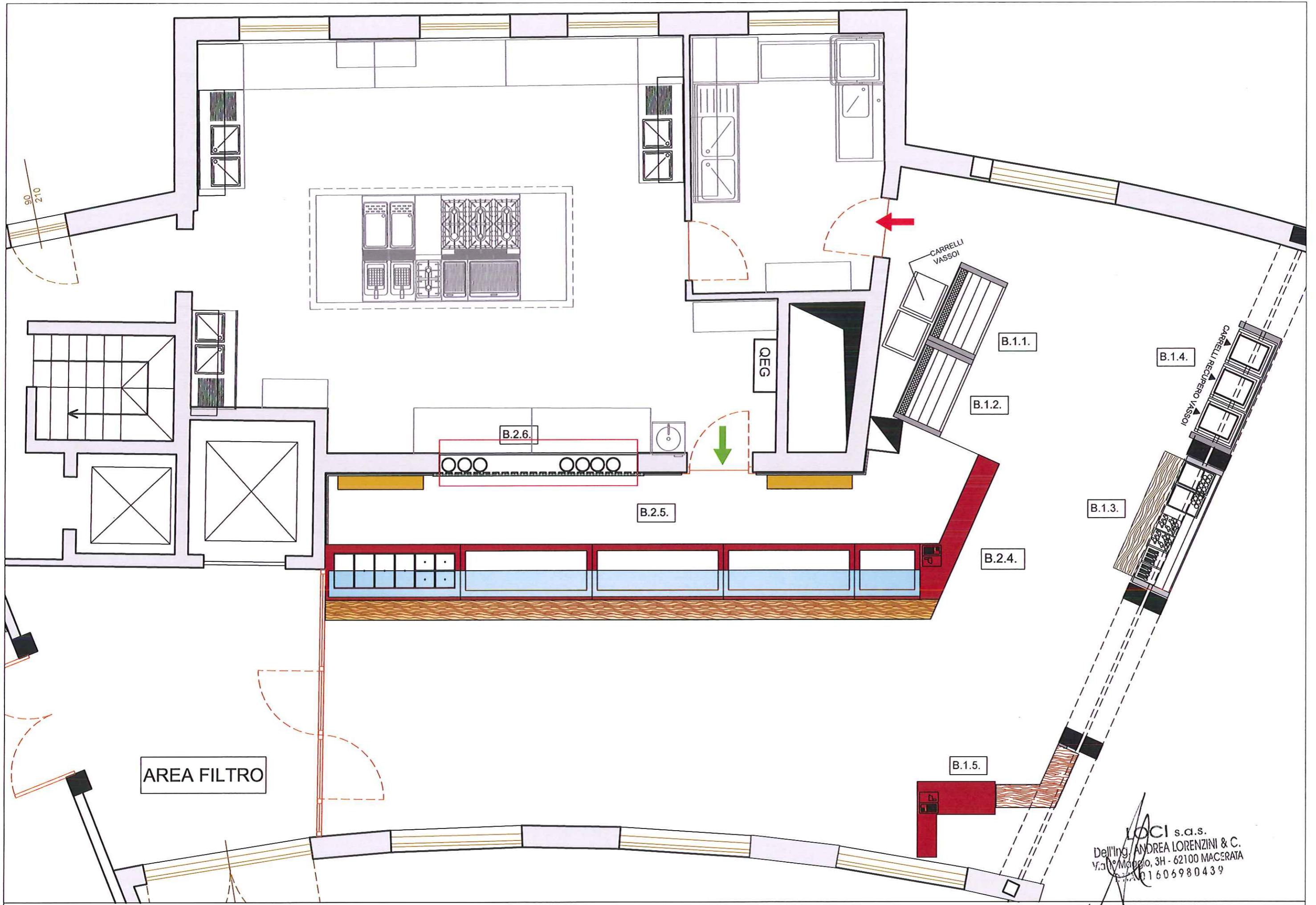
TAV. 03-01 SELF SERVICE PLANIMETRIA TOTALE 04/09/2015 scala 1:50
