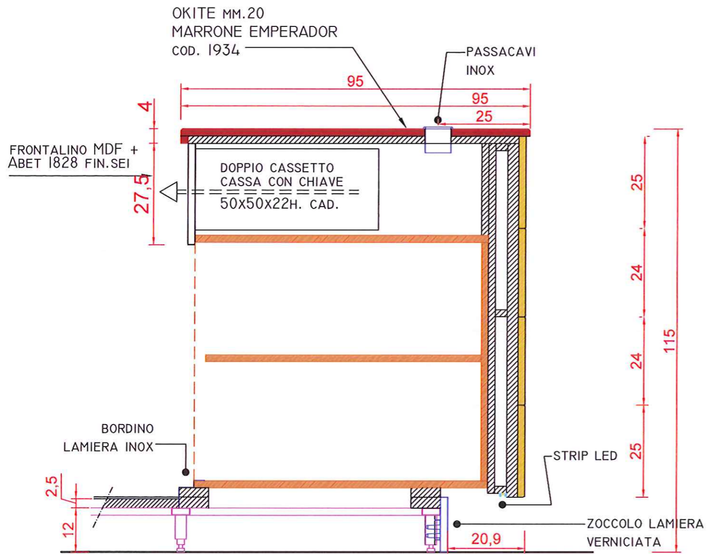
SEZIONE AA': BANCO CASSA
