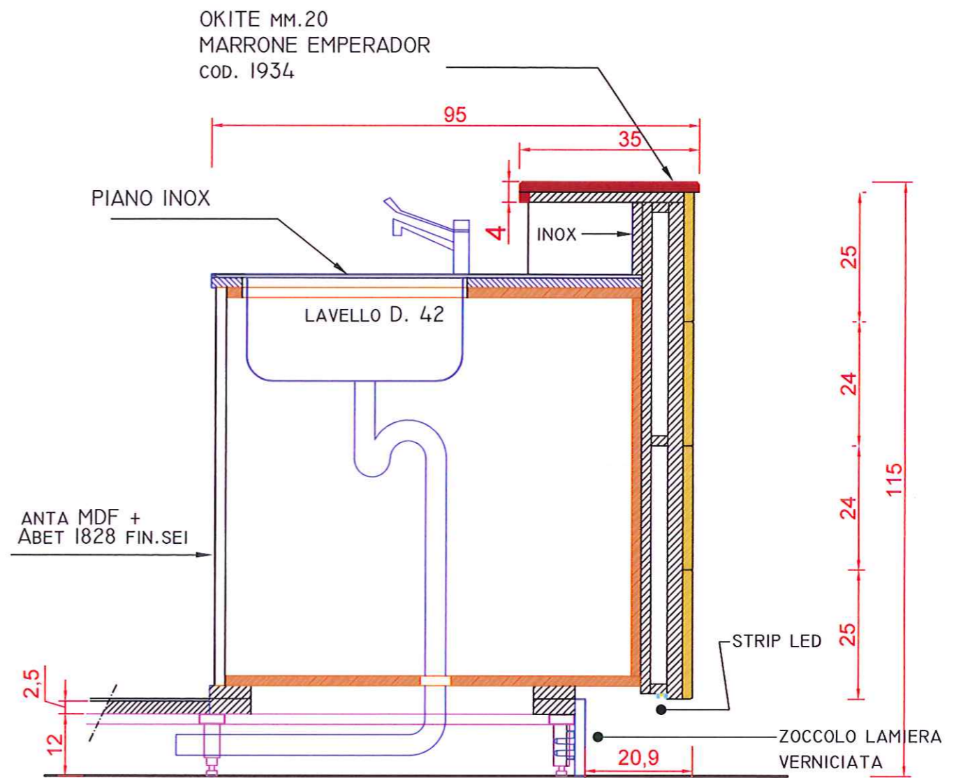
SEZIONE BB': BANCO LAVELLI
