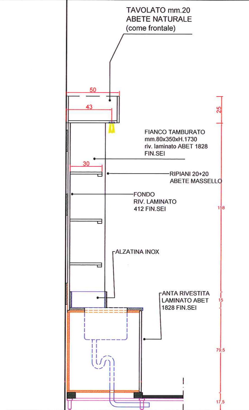
SEZIONE FF': RETRO LAVELLO
