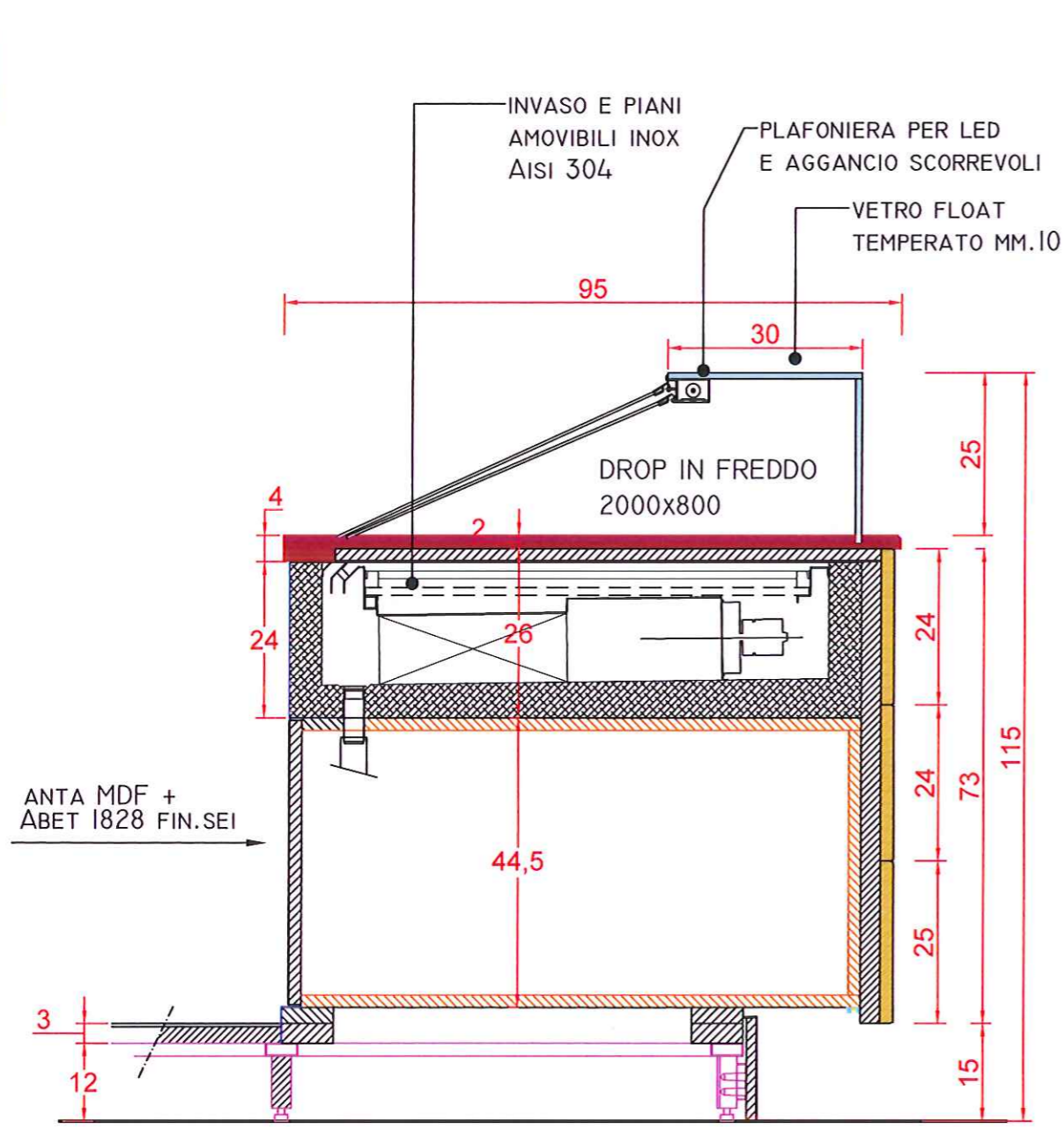
SEZIONE DD': VETRINA FREDDA
